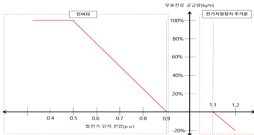
<고장발생 후 무효전류 공급능력>
