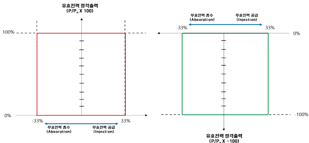
<유효전력 출력에 따른 무효전력 공급범위>
