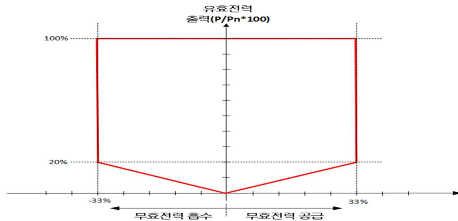
<유효전력 출력에 따른 무효전력 공급범위>
